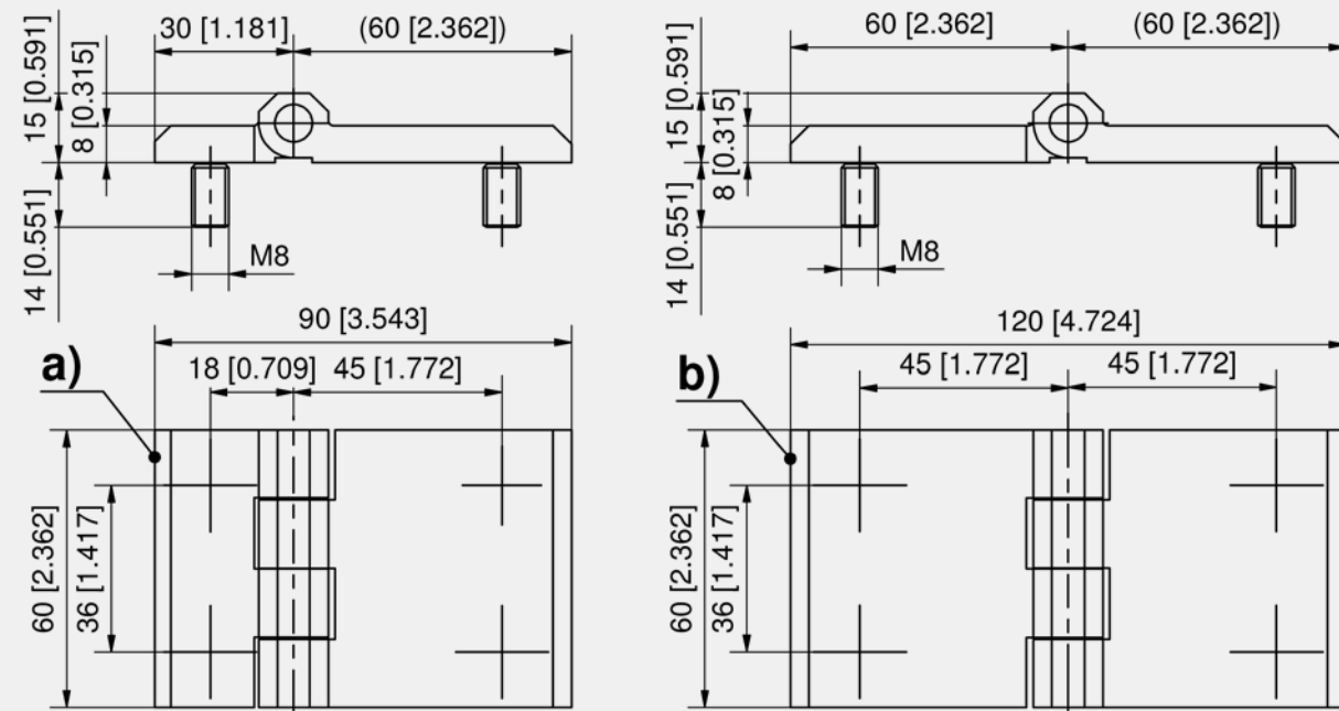
Hinge, zinc die
