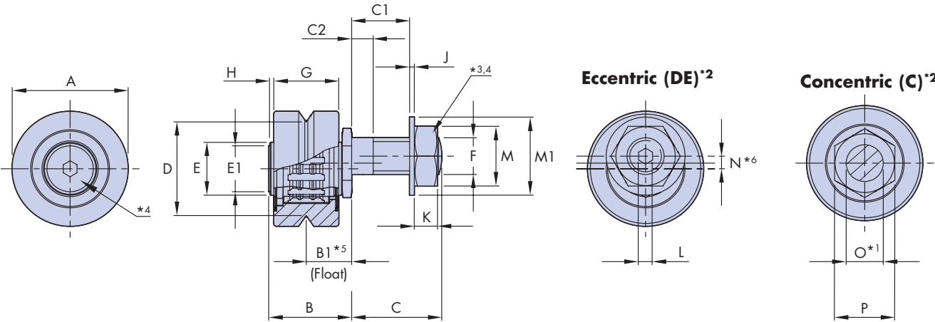
Short stud (RSFJ) / Long stud (RLFJ)
