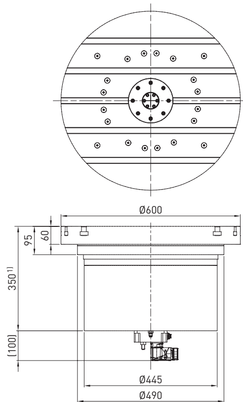
RCH-600 dimensions
