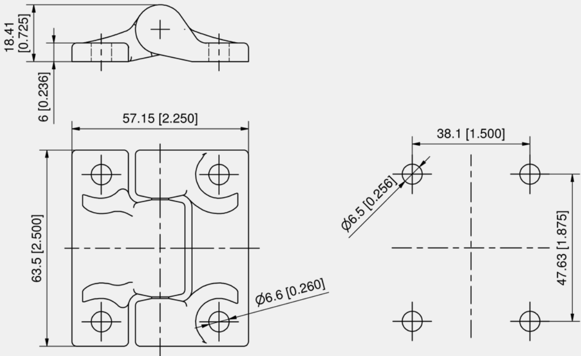
Torque hinge
