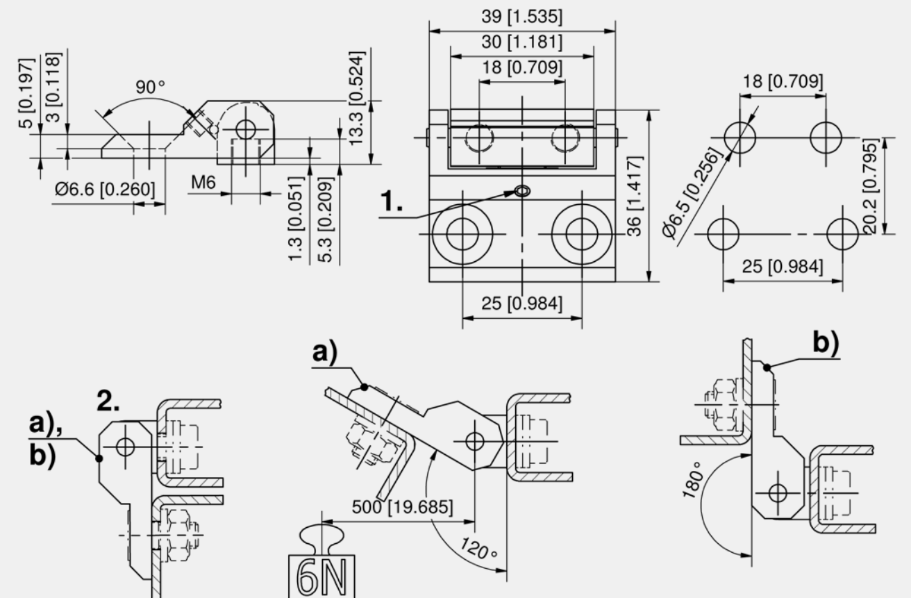
Detent hinge
