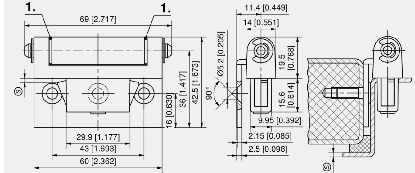
Hinge
