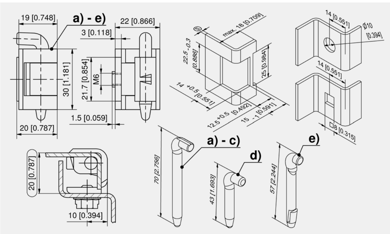
Hinge
