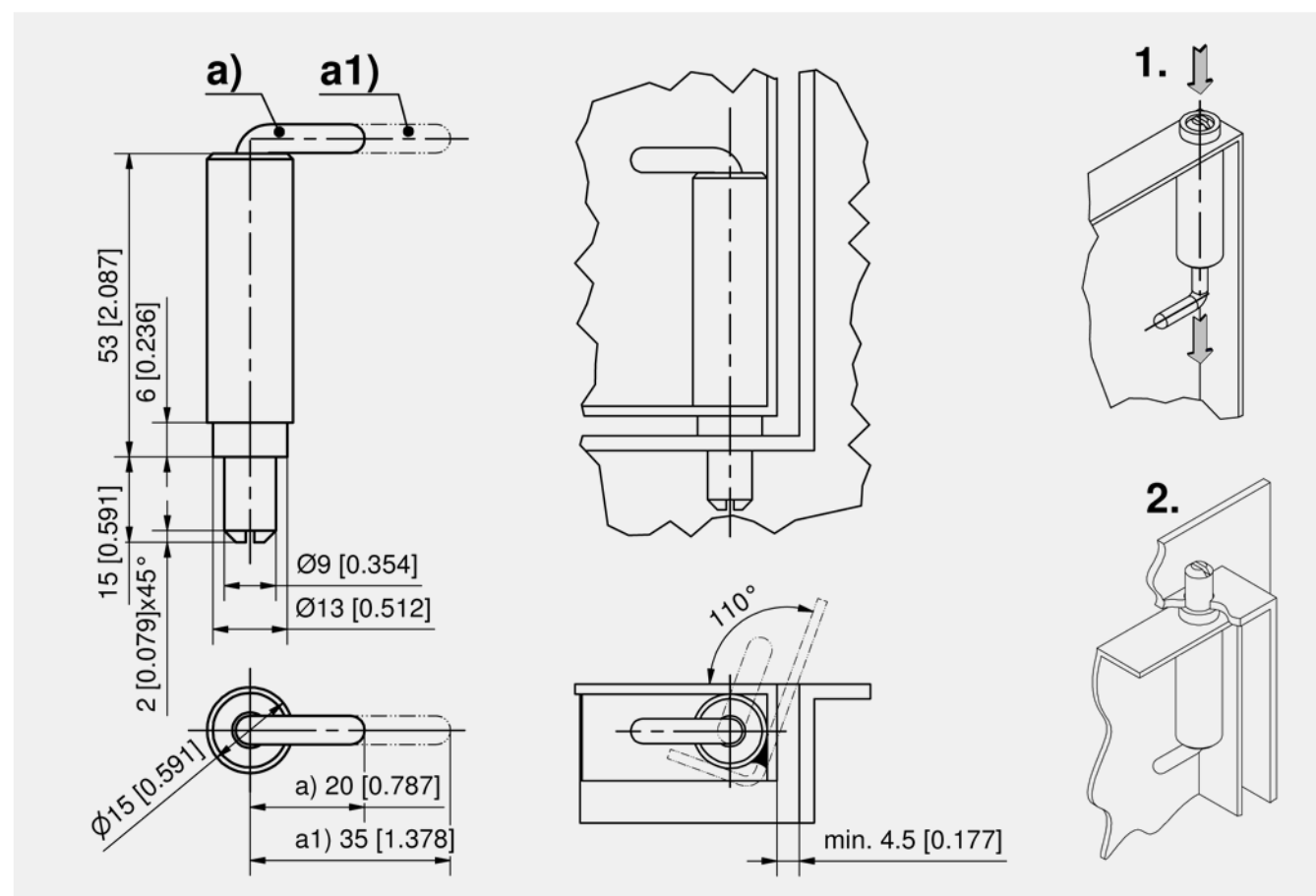
Pin hinge
