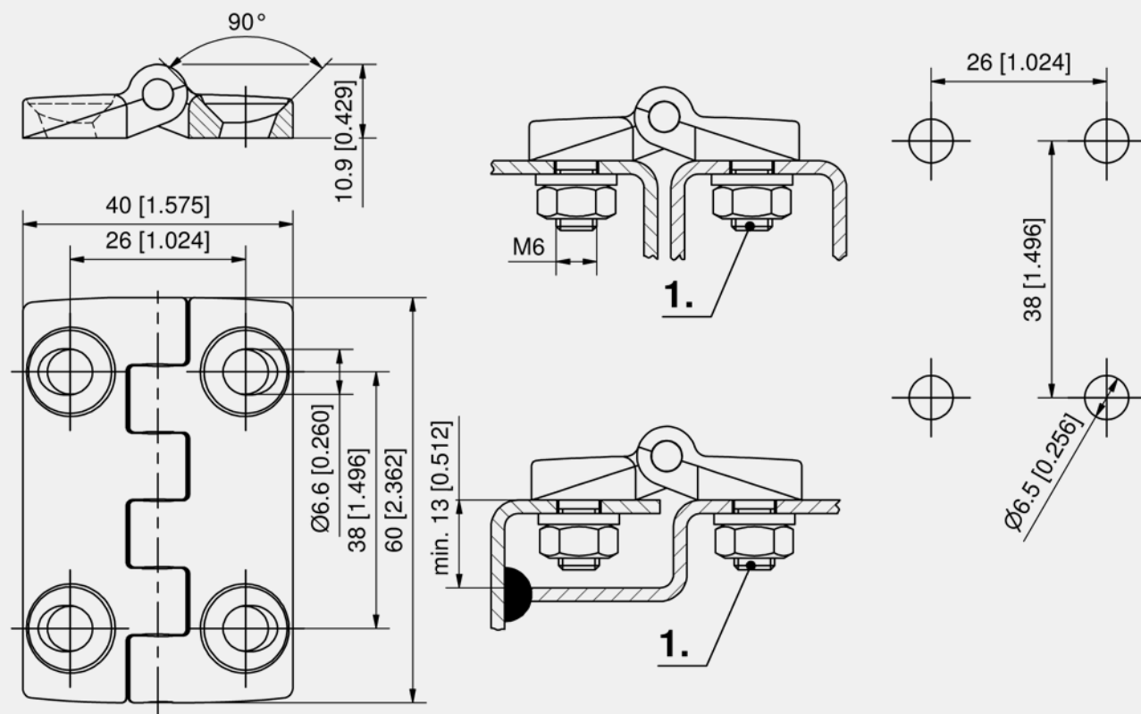
Hinge
