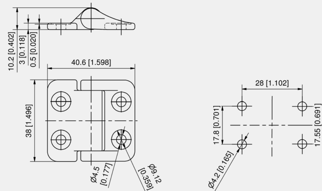
Torque hinge
