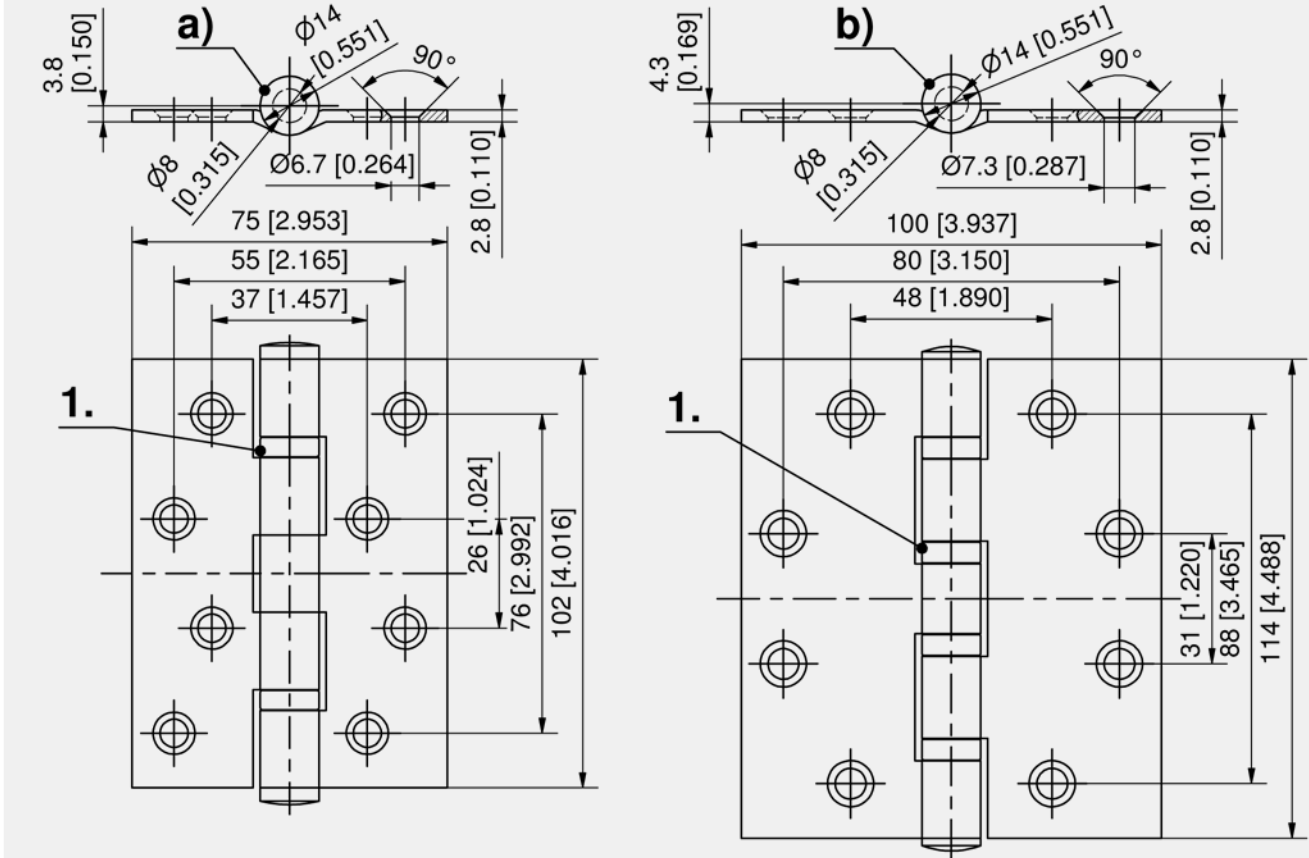
Hinge
