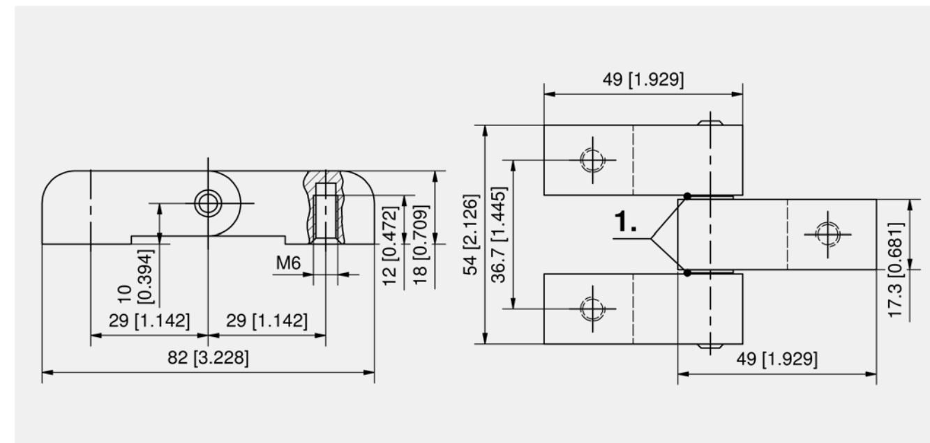
Hinge
