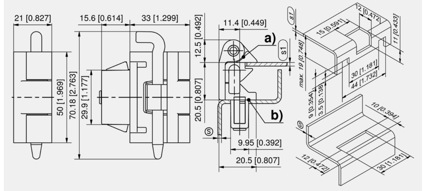
Hinge
