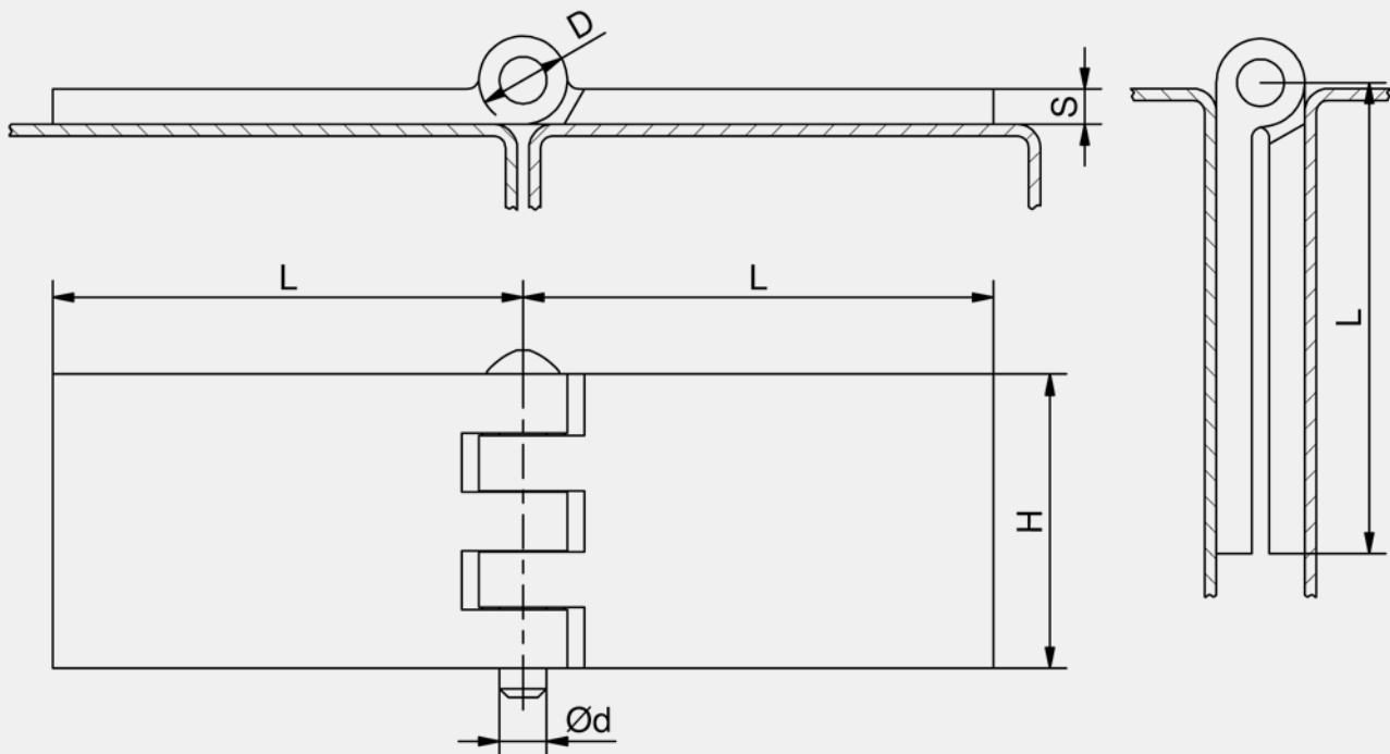
Hinge
