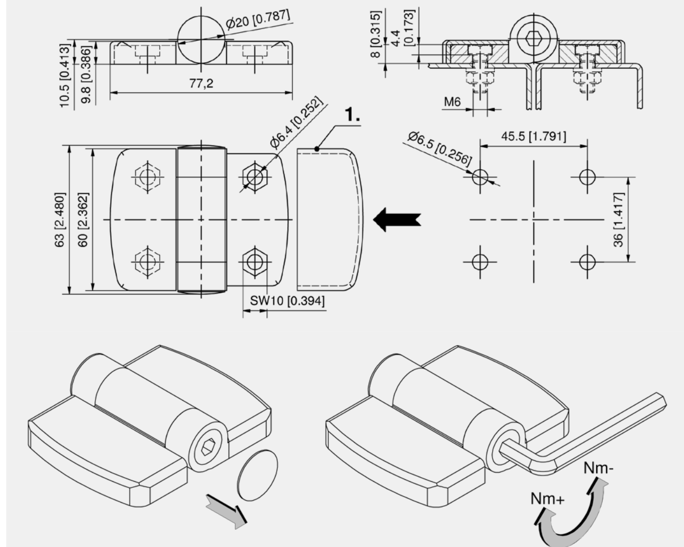
Torque hinge
