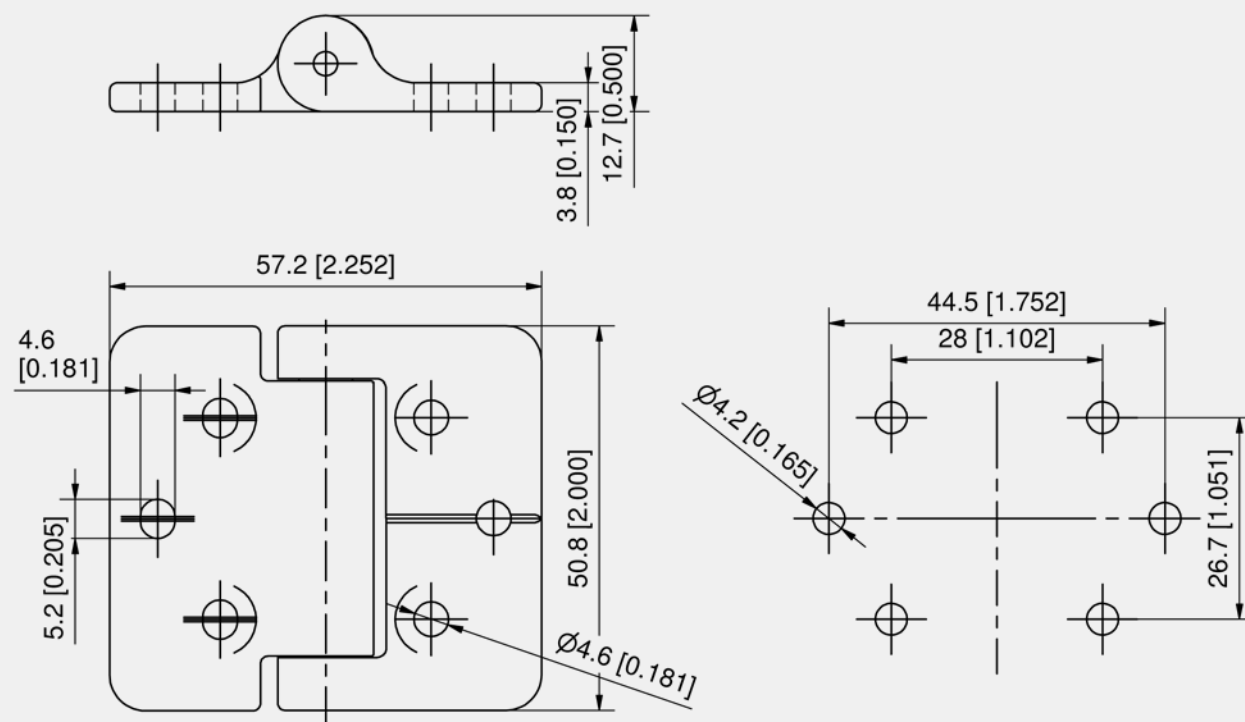
Torque hinge
