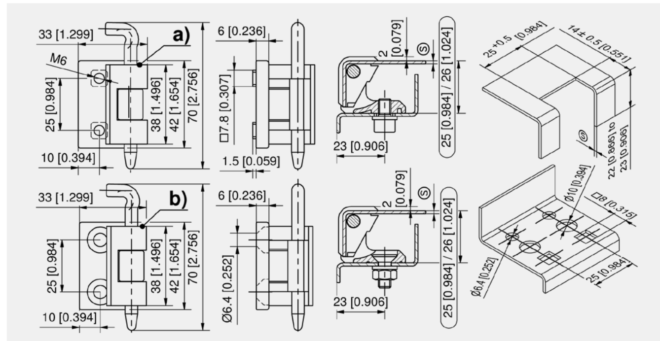
Hinge
