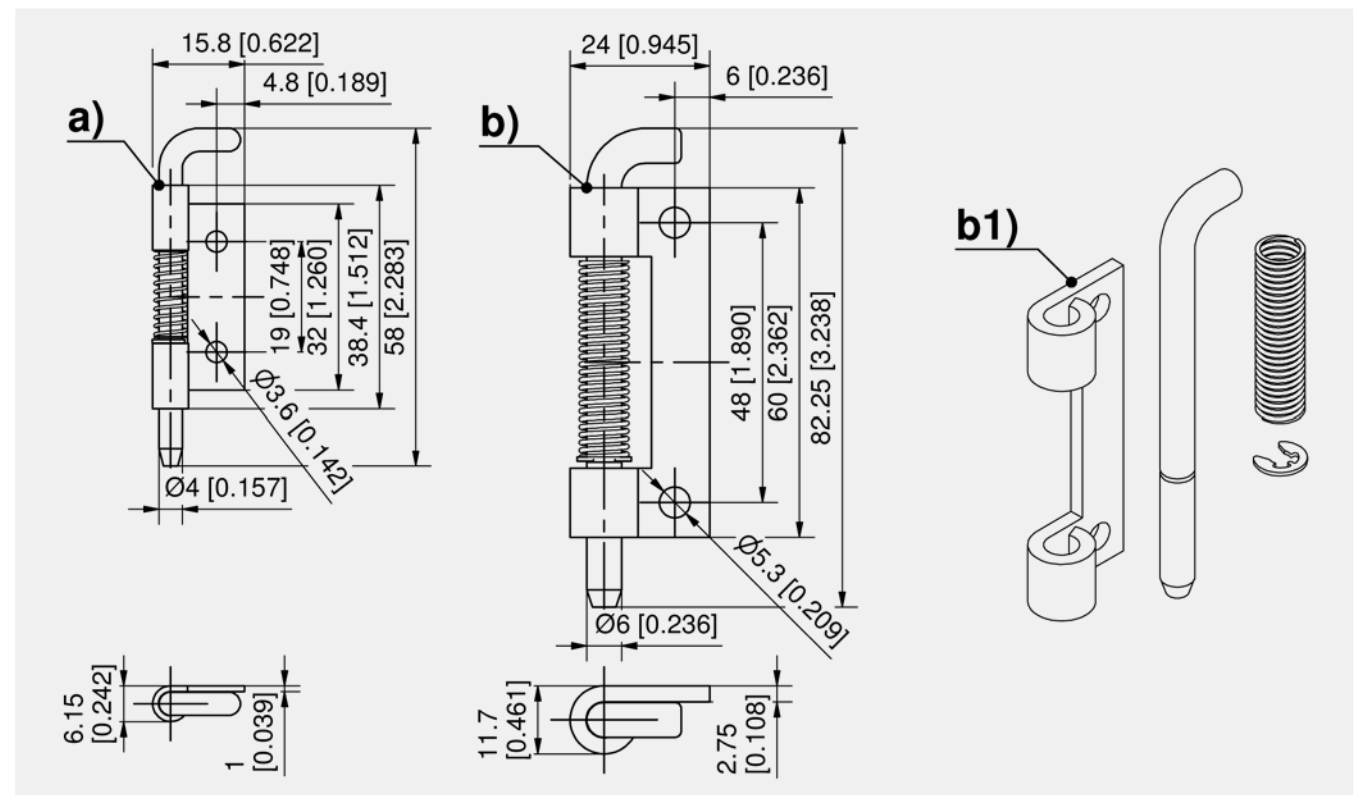
Pin hinge
