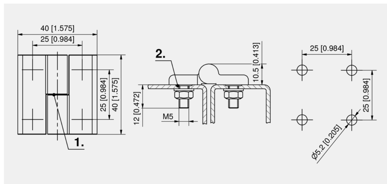
Hinge
