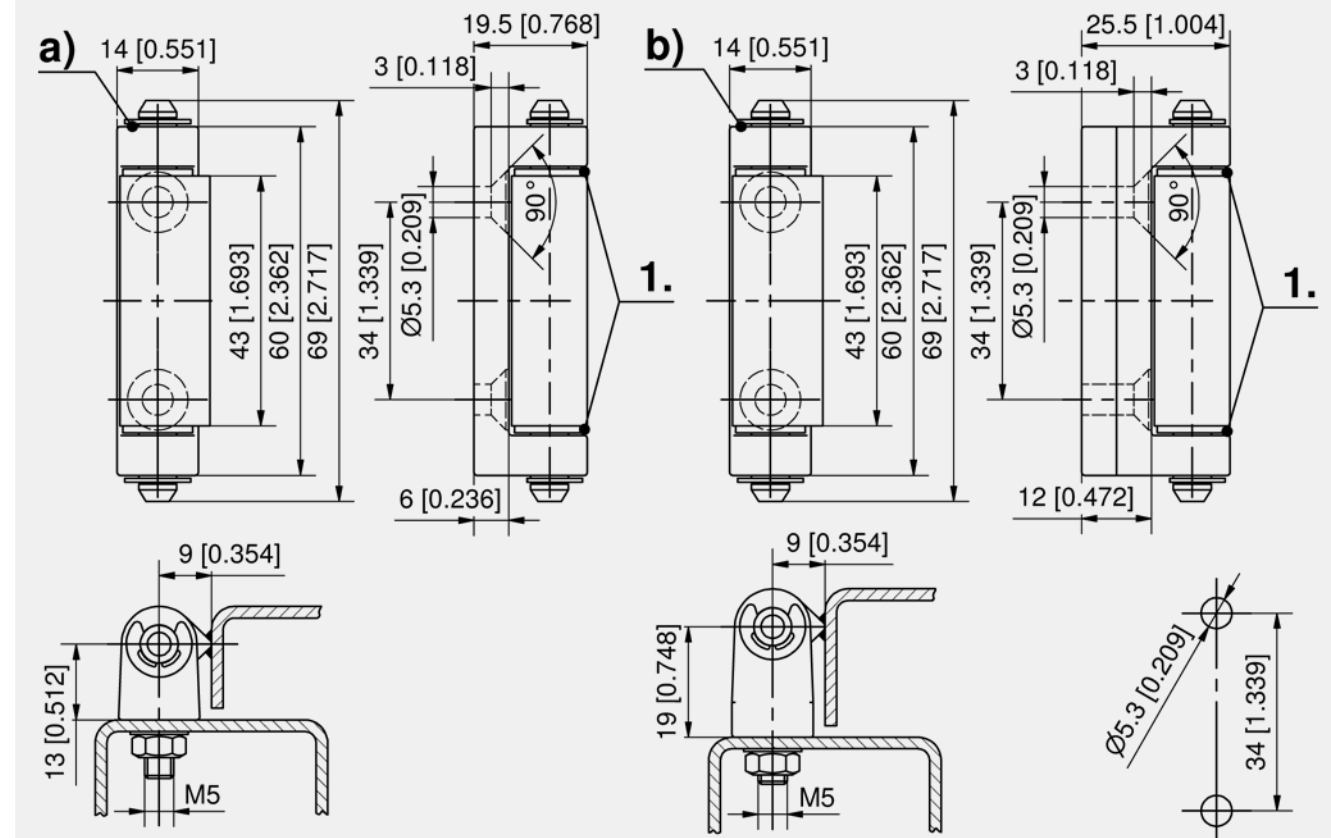
Corner hinge, zinc die
