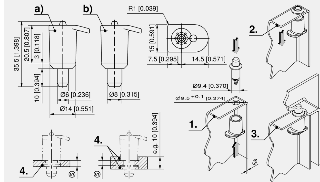
Pin hinge
