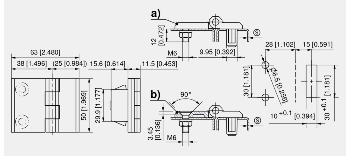
Hinge
