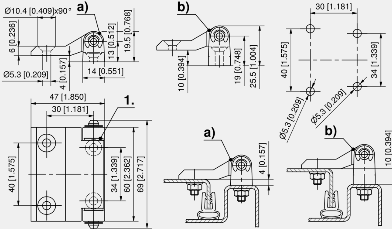
Hinge
