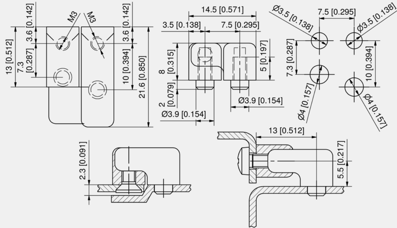
Hinge
