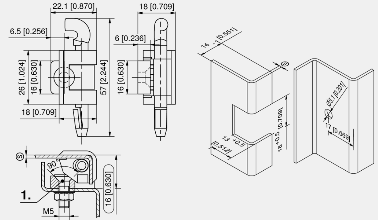
Hinge
