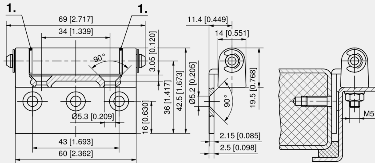
Hinge
