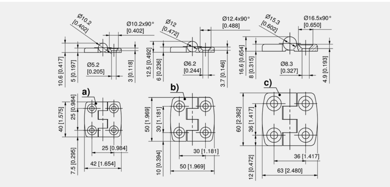
Hinge
