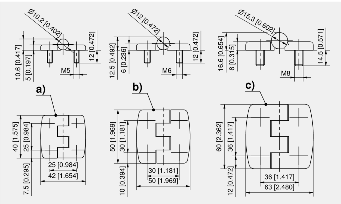
Hinge
