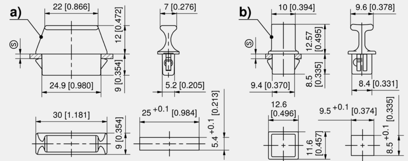
Grip handle, zinc die
