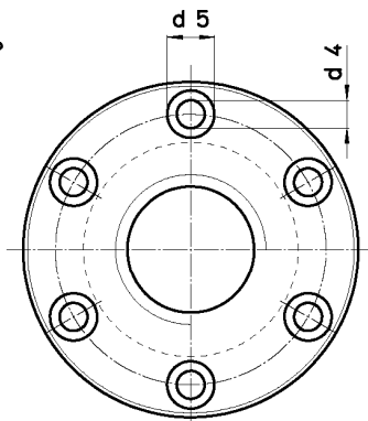
Od Tr 25x5 (6 rupa)
