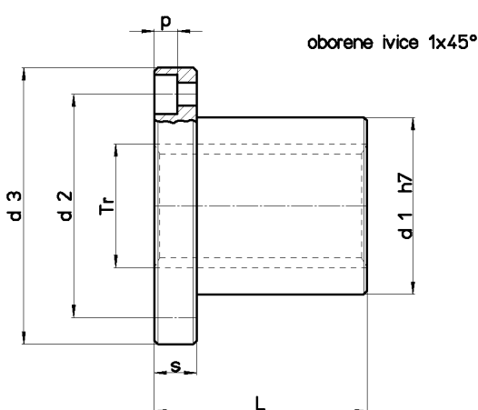
Od Tr 25x5 (6 rupa)
