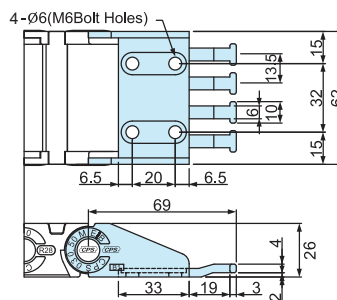
CPS030.50 Punto mobile
