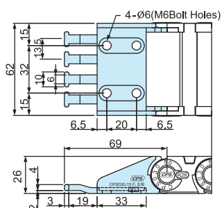
CPS030.50 Punto fisso
