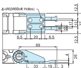
CPS030.25 Punto mobile
