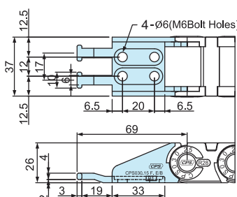
CPS030.25 Punto fisso
