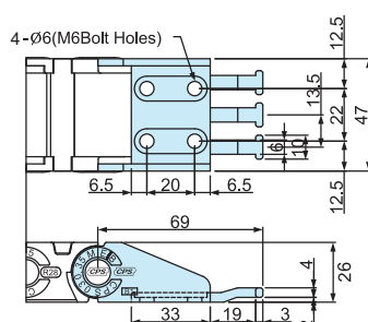
CPS030.35 Punto mobile
