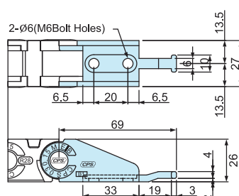
CPS030.15 Punto mobile
