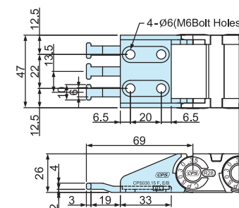
CPS030.35 Punto fisso
