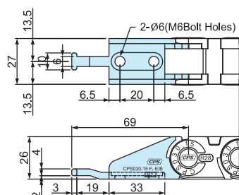
CPS030.15 Punto fisso
